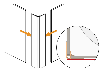
Eckprofil, innen/Profilé d'angle intérieur Bei Sanierung empfohlen. Recommandé pour la rénovation.
