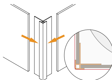
Eckprofil, außen/Profilé d'angle extérieur Bei Neueinbau empfohlen. Recommandé pour les nouvelles constructions.
