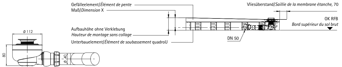
Einbau waagerechter Ablauf/Montage écoulement horizontal
