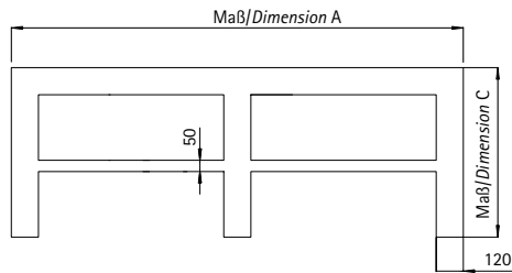
Ansicht von vorn/Vue de face
