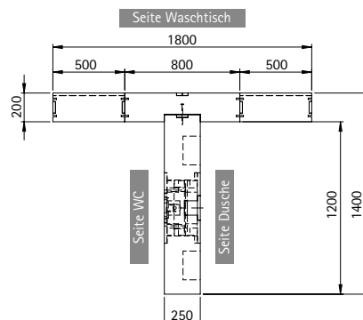
Draufsicht/Vue de dessus
