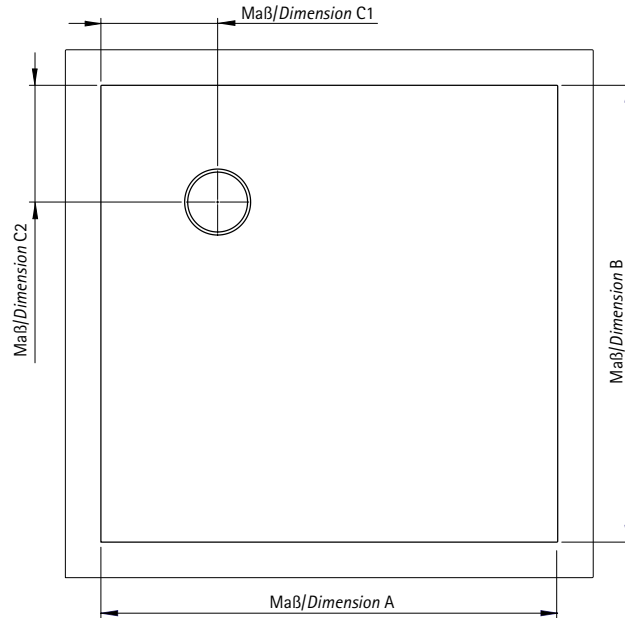
Allgemeine Draufsicht/Vue générale de dessus PLAN PLUS ROUND 20
