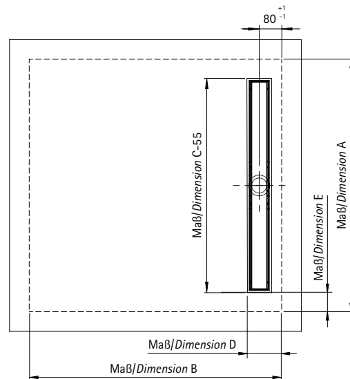
Allgemeine Draufsicht/Vue générale de dessus LINE2FR
