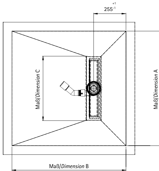
Allgemeine Draufsicht/Vue générale de dessus LINE PLUS PURE
