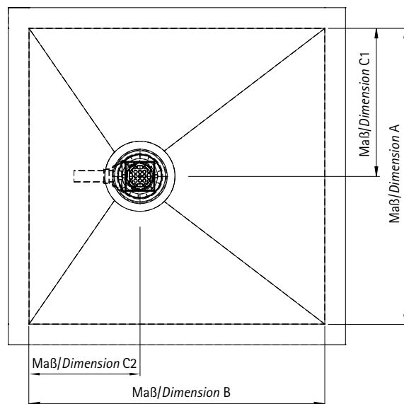
Allgemeine Draufsicht/Vue générale de dessus LEVEL 18
