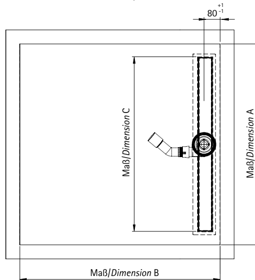
Allgemeine Draufsicht/Vue générale de dessus LINEPLUS PURE
